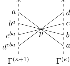
FIGURE 4. Actual vertex
